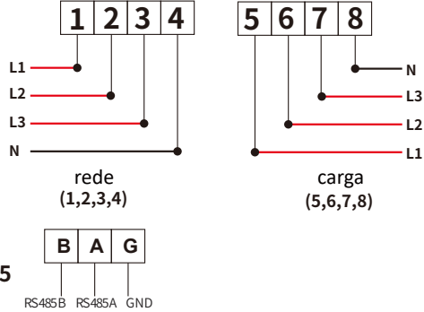
Figura 7.20 Medidor Eastron
