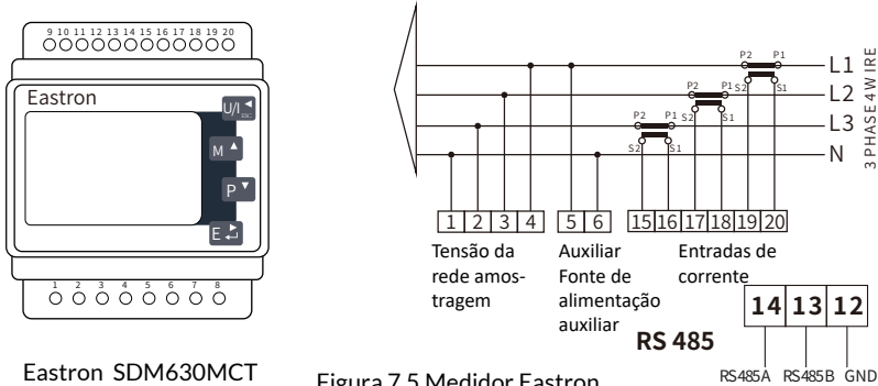
Figura 7.5 Medidor Eastron
